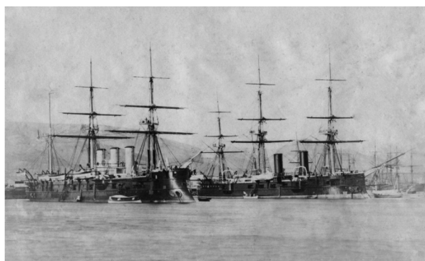
Рис. 1. Греция. 1890. Броненосный крейсер «Память Азова» и полуброненосный фрегат «Владимир Мономах» в Пирее
